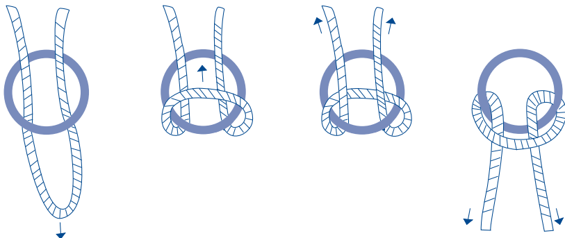
ankersteek
